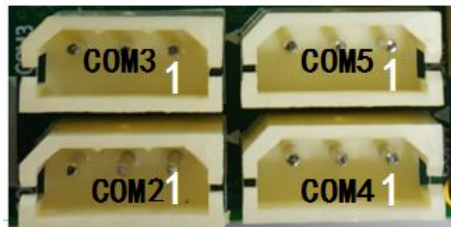
1x3PIN2.5mm 间距 180 度 wafer 座子
