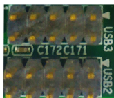
2 个 2*5PIN 2.0mm 间距 180度排针
